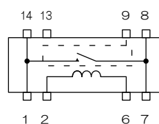
DIP-1M-※※S
