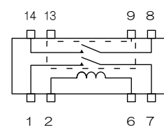
DIP-2M-※※S
