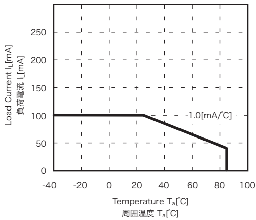
Load Current vs. Temperature 負荷電流-周囲温度特性
