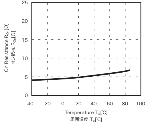
On Resistance vs. Temperature オン抵抗-周囲温度特性 ( I_F=5[mA] , I_L=100[mA] )
