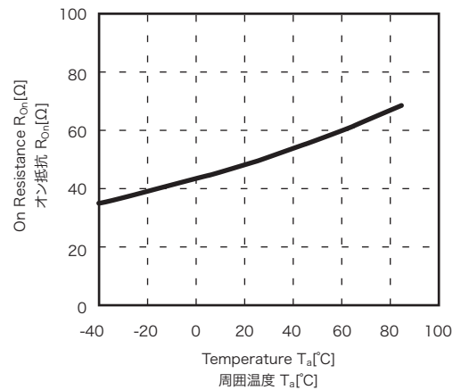
On Resistance vs. Temperature オン抵抗-周囲温度特性 ( I_F=5[mA] , I_L=10[mA] )
